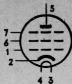
Miniatur B7G
